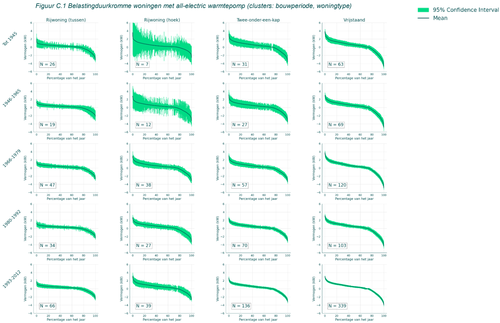
Figuur C.2 Belastingduurkromme (elektrisch) woningen met all-electric warmtepomp (clusters: bouwperiode, verliesoppervlak) Legend: 95% Confidence Interval (green shaded area), Mean (black line).
