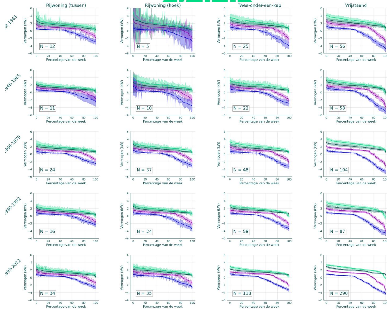
Figuur C.3 Belastingduurkromme van all-electric warmtepompen over vier referentiweeken (woningtype, bouwperiode)
