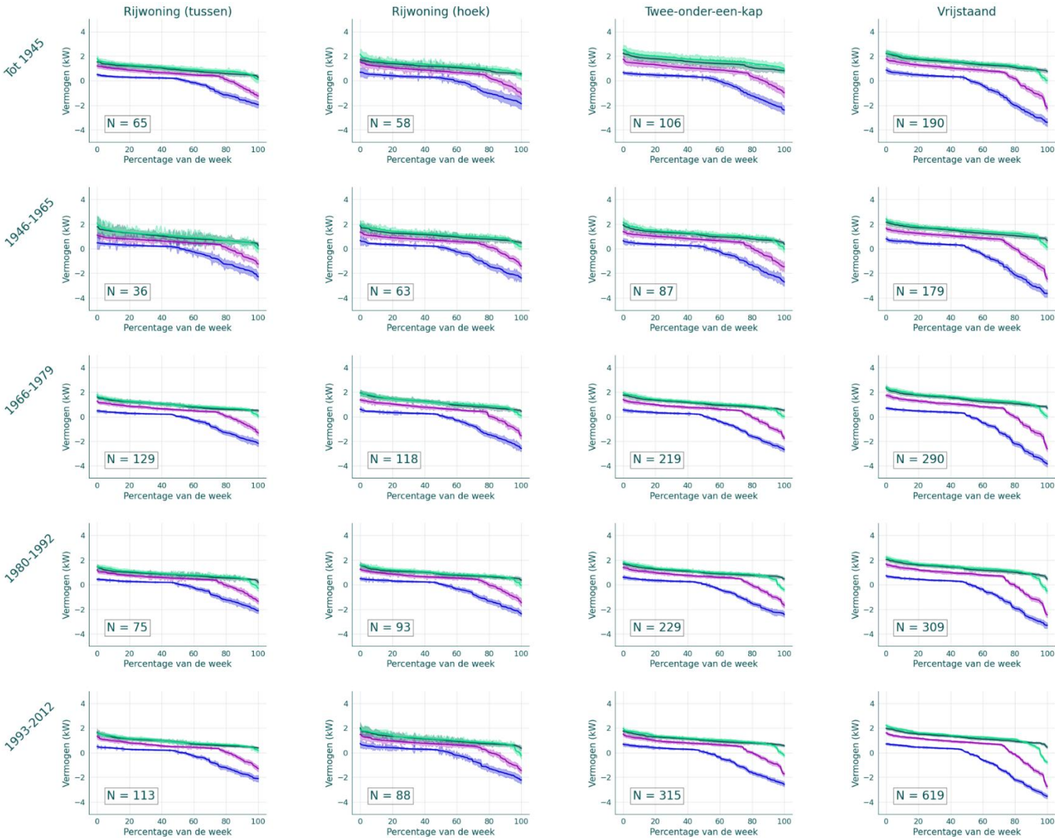
Figuur B.3 Belastingduurkromme referentieweken woningen met hybride warmtepomp (clusters: bouwperiode, woningtype)
